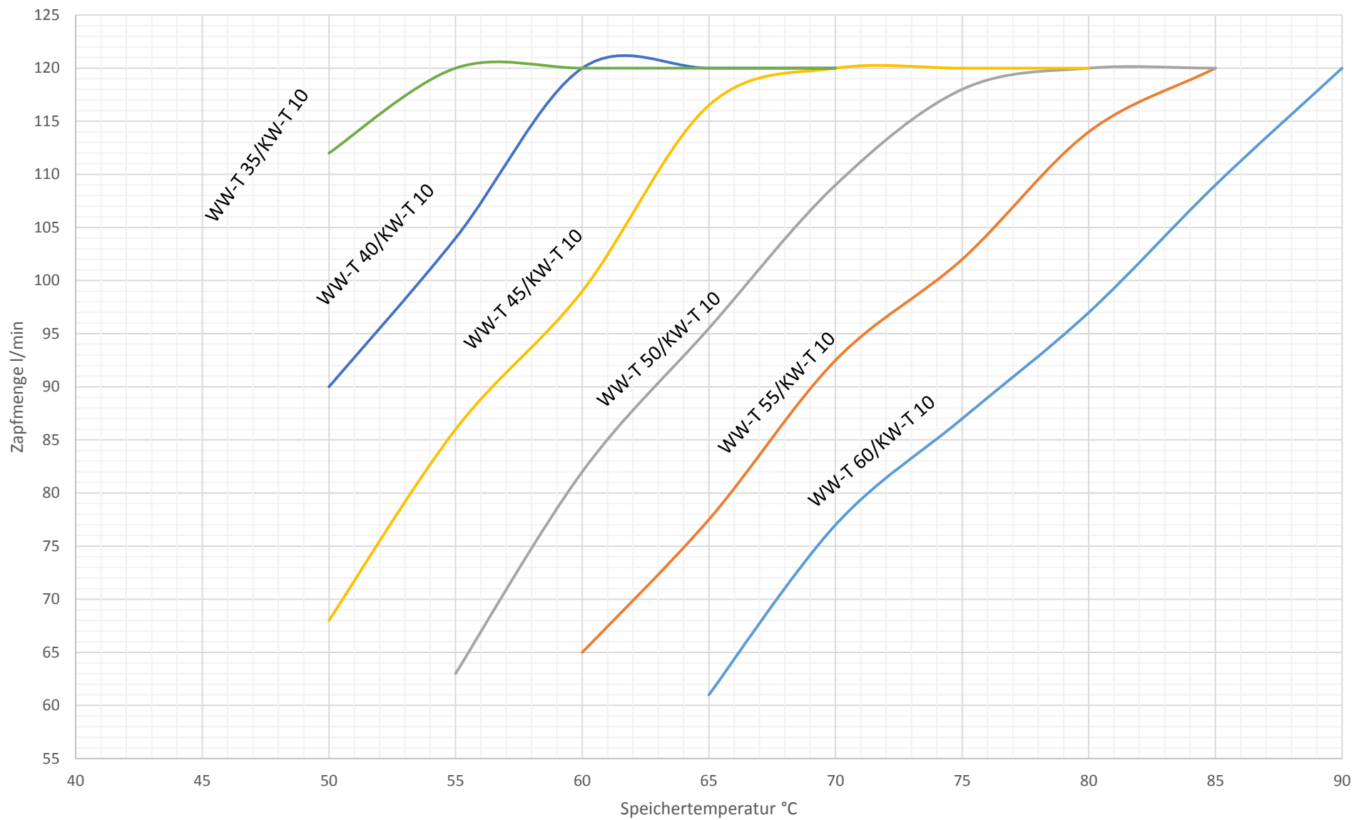
Auslegungsdiagramm 3er Kaskade
